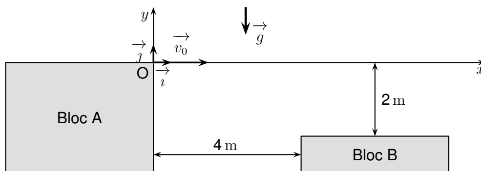
Figure 1 : schématisation des conditions du saut
